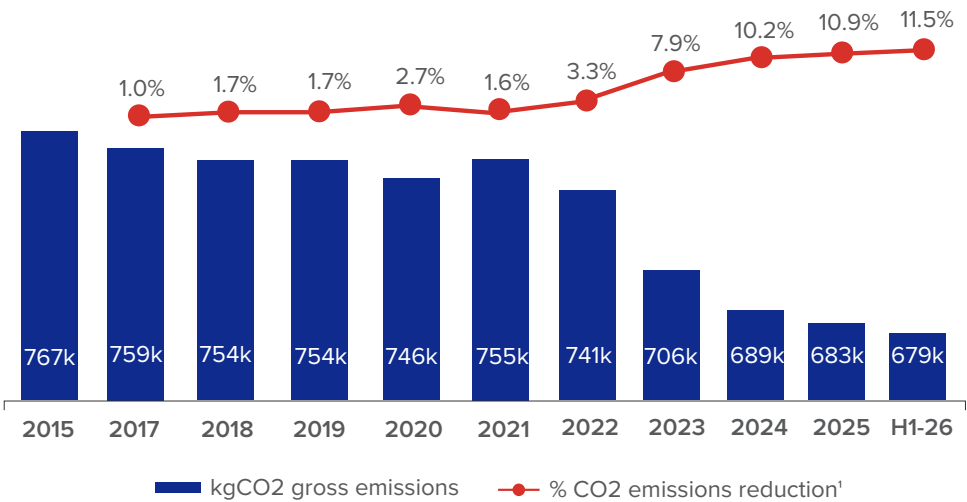
CO2 EMISSIONS
